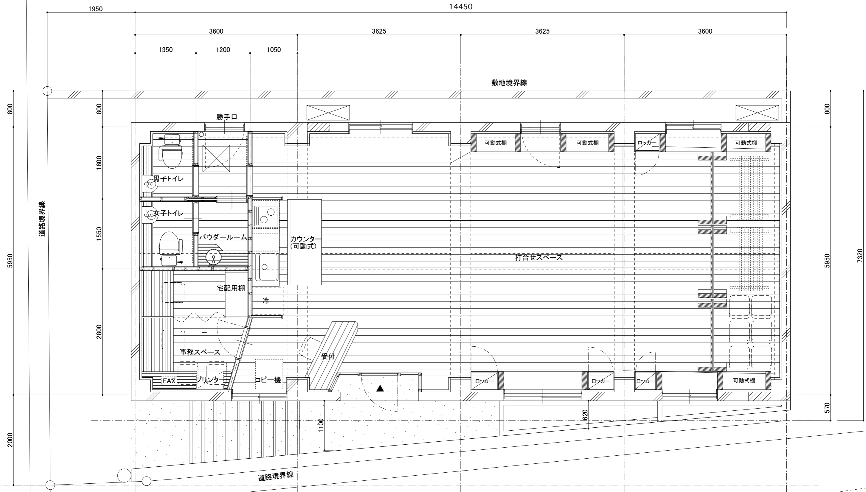
スタジオレイアウト
